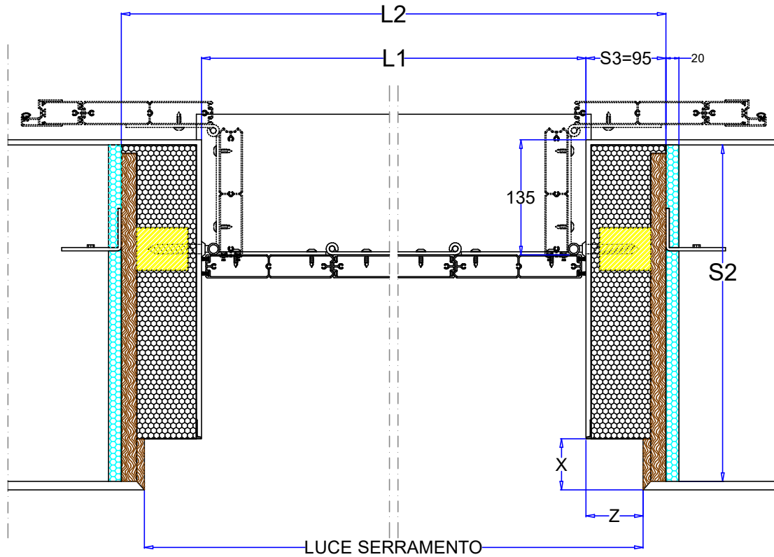
S e z i o n e O r i z z o n t a l e
