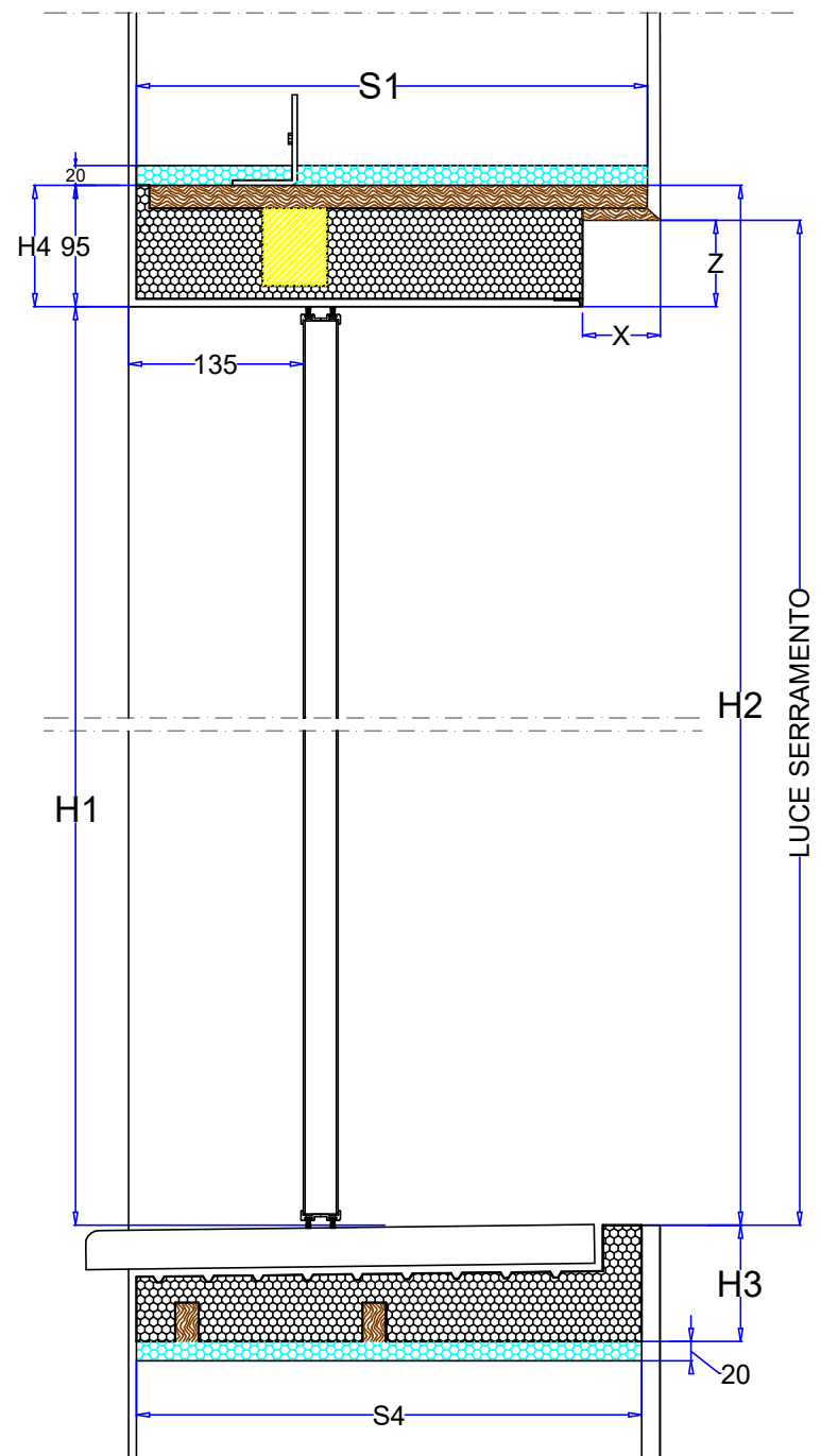
S e z i o n e V e r t i c a l e
